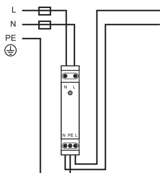
Conexión en serie Series connection Connexion en série
