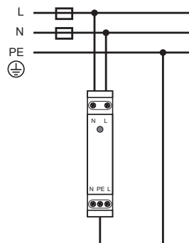
Conexión en paralelo Parallel connection Connexion en parallèle
