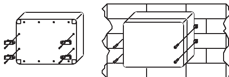
Detalle colocación Garras
