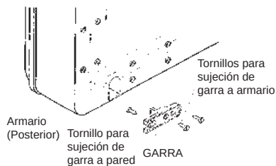
Detalle colocación Garras
