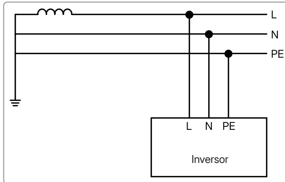
Figura 4-4 TN-S
