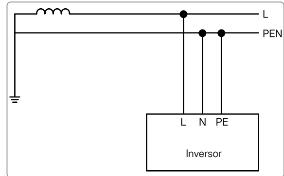
Figura 4-5 TN-C
