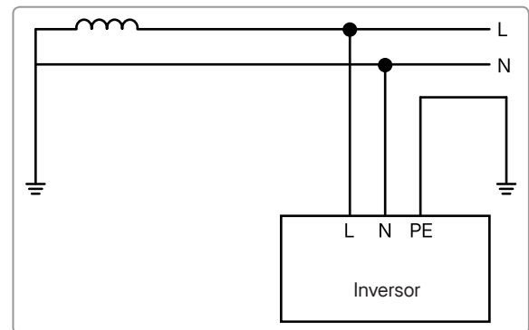
Figura 4-7 TT
