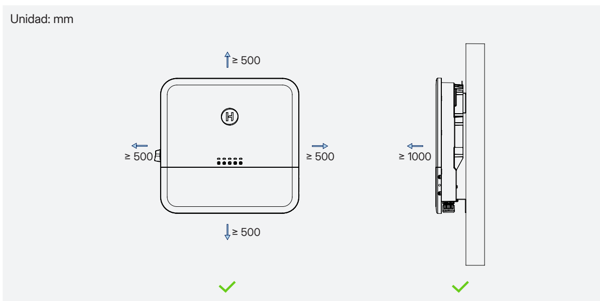
Figura 6-2 Instalación correcta
