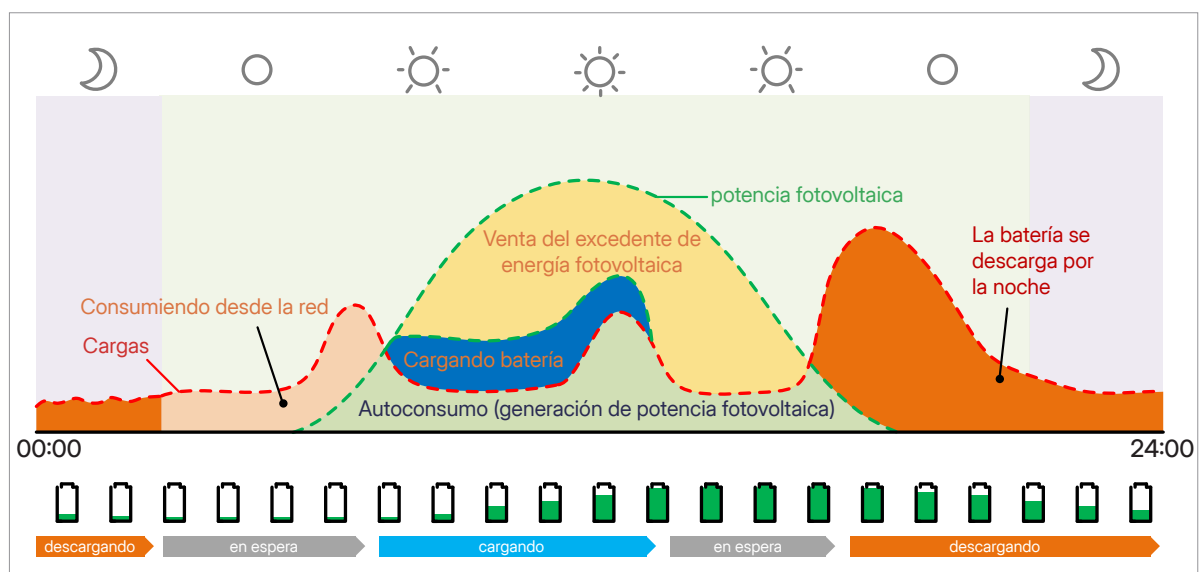
Figura 4-8 Flujo de energía del modo de autoconsumo
