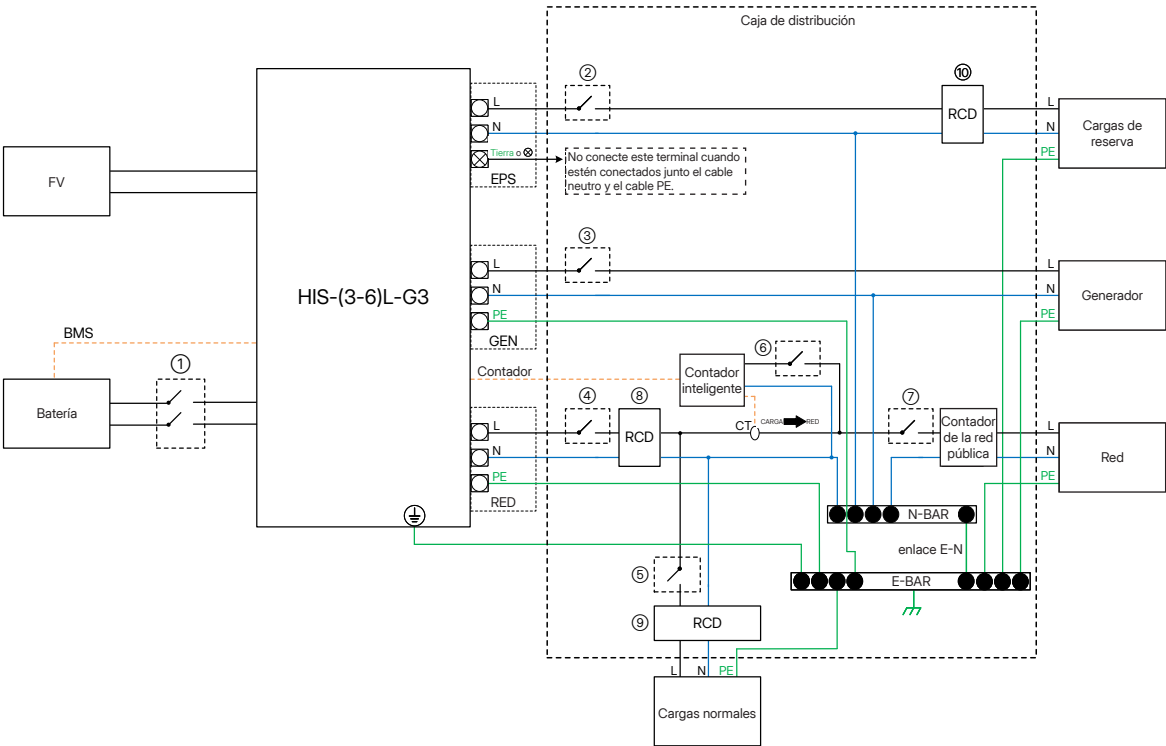
Figura 7-1 Diagrama básico 1
