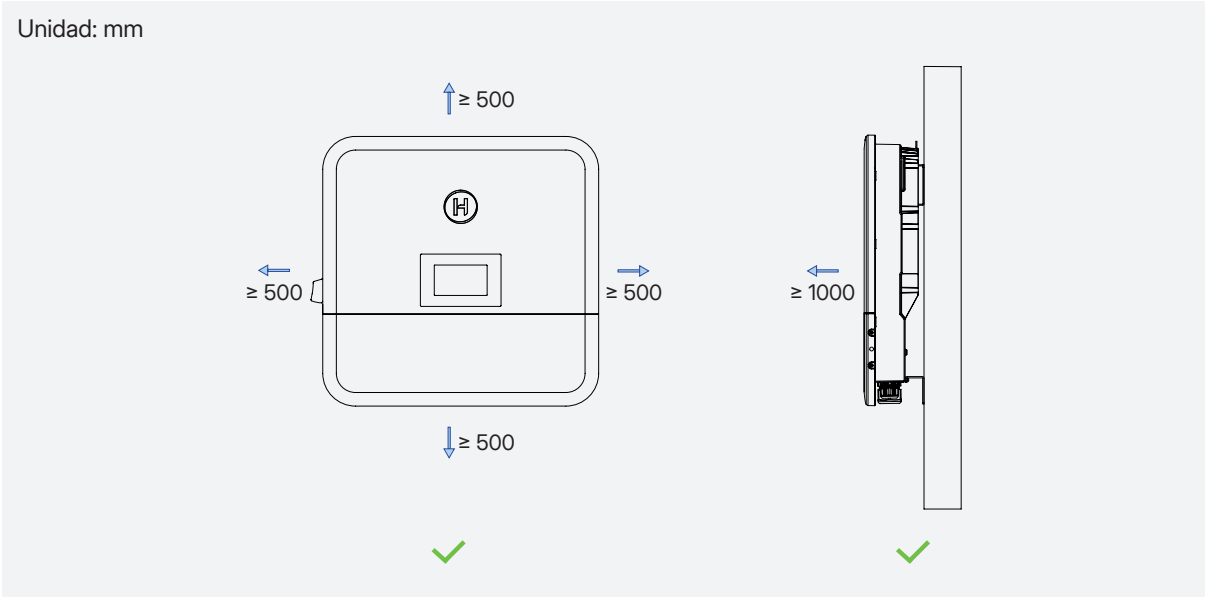
Figura 6-2 Instalación correcta
