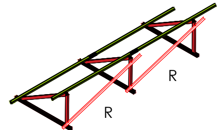
Disposición de los arriostramientos A08 para montajes de 3 pórticos
