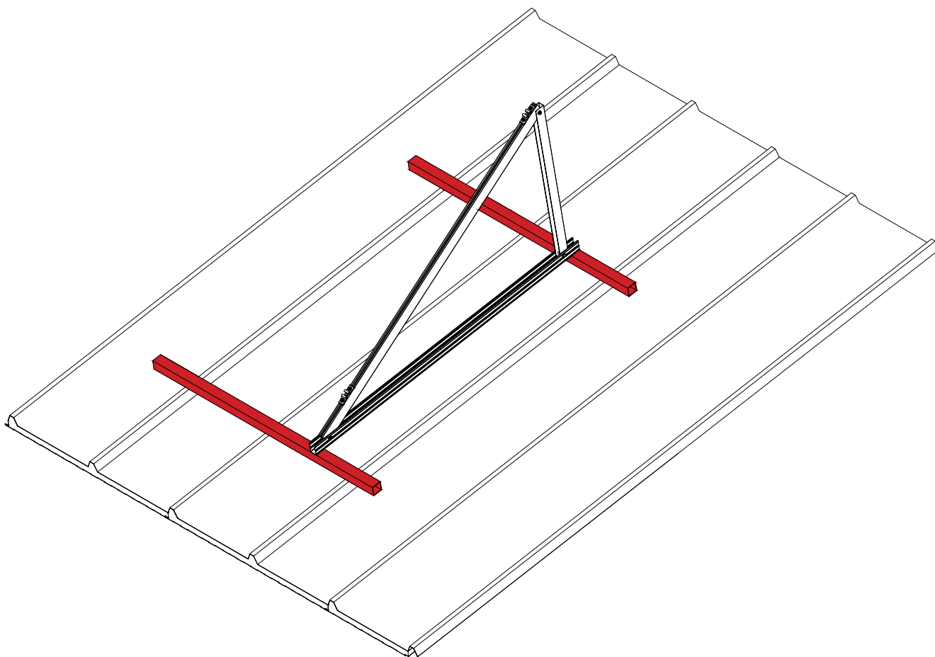
Ejemplo subestructura
