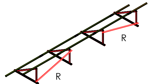
Disposición de los arriostramientos A08 para montajes de 4 o más pórticos
