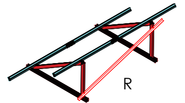
Disposición de los arriostramientos A08 para montajes de 2 pórticos
