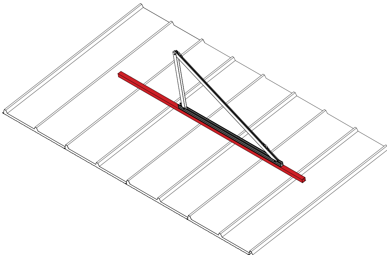
Ejemplo subestructura
