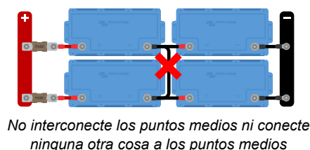
Varias baterías en serie/paralelo
