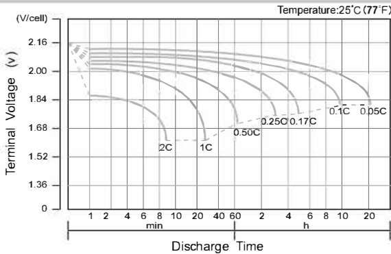
Características de la curva de descarga
