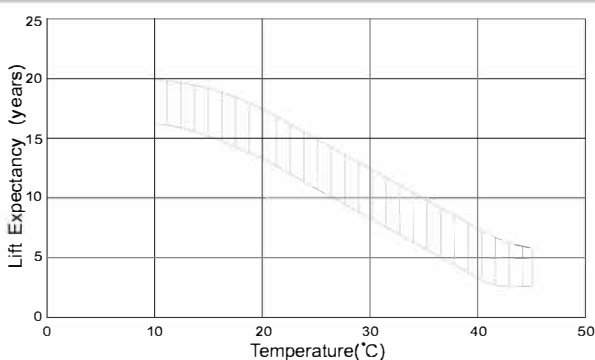
Efectos de la temperatura en la vida a largo plazo
