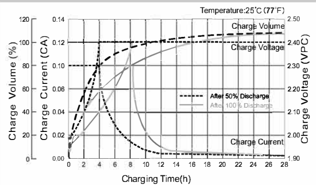
Características de la curva de carga por ciclo de uso (IU)
