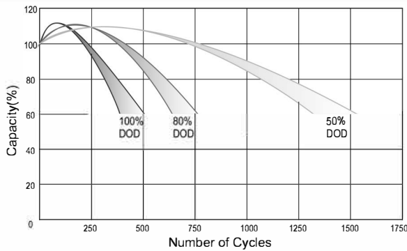
Ciclos de vida en función de la profundidad de descarga
