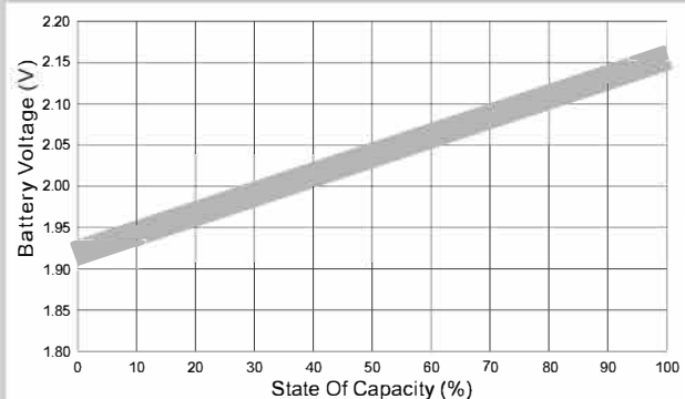
Relación entre OCV y el estado de carga (20°C)
