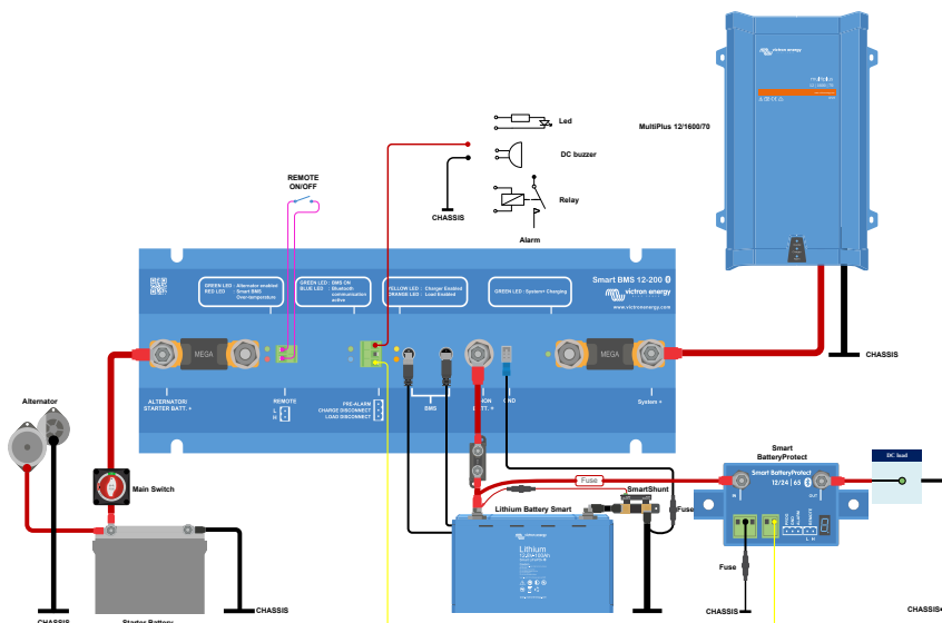
Ejemplo de aplicación con MultiPlus y Smart BatteryProtect
