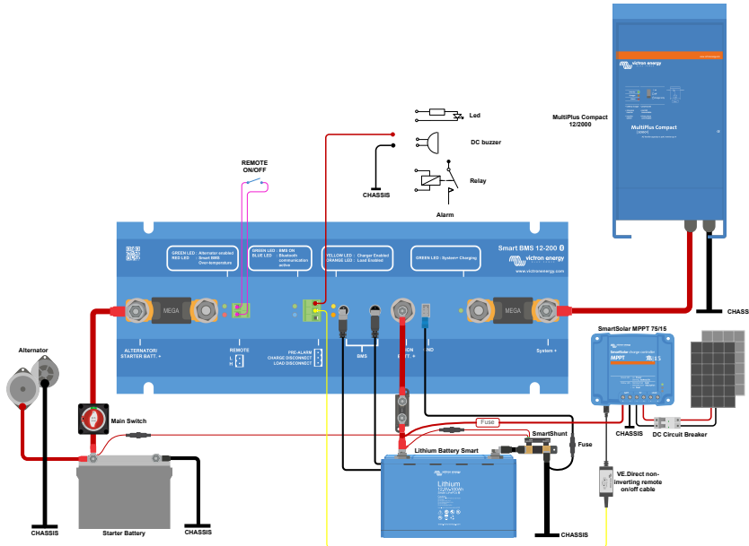
Ejemplo de aplicación con un MultiPlus Compact y un MPPT
