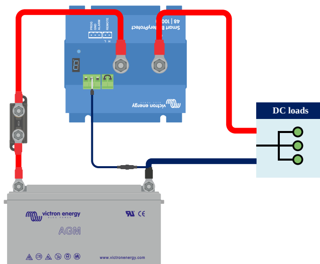
Smart BatteryProtect en un sistema sencillo con puente entre la entrada L y H (predeterminado de fábrica)
