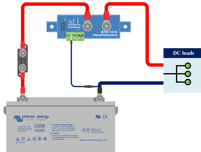
Smart BatteryProtect en un sistema sencillo con puente entre la entrada L y H (predeterminado de fábrica)
