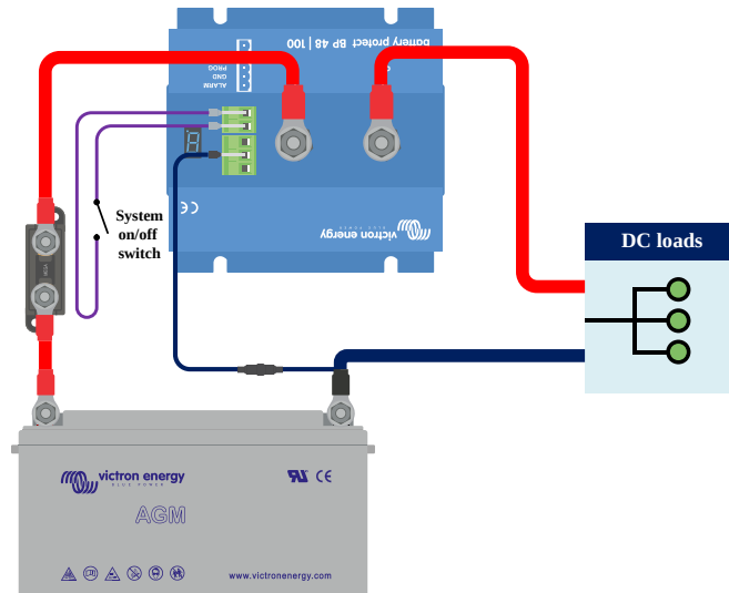
BatteryProtect con interruptor on/off remoto
