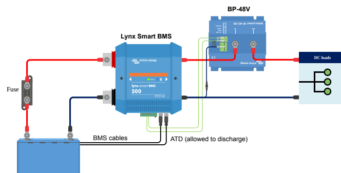
BatteryProtect en modo Li-ion controlado por ATD (permitir la carga) desde un Lynx Smart BMS
