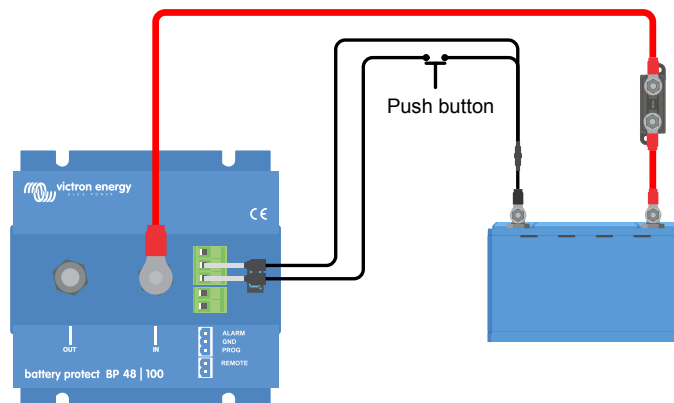
Pulsador conectado para programar el BatteryProtect
