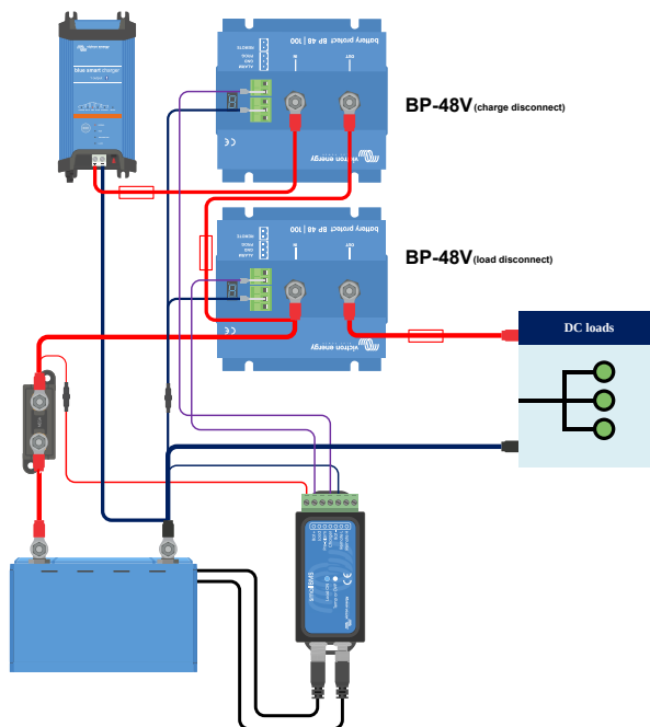
Dos BatteryProtect toman el control de un cargador y un circuito de cargas
