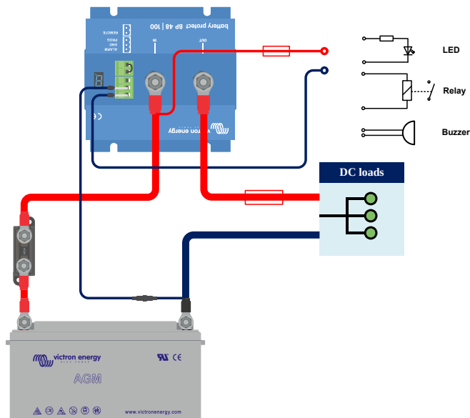
Conexión de un LED, una señal acústica o un relé a la salida del BatteryProtect
