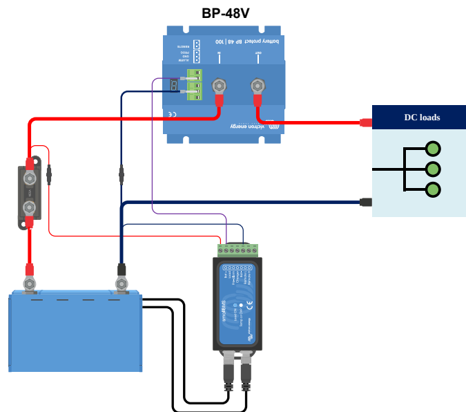
BatteryProtect usa la desconexión de las cargas de un smallBMS
