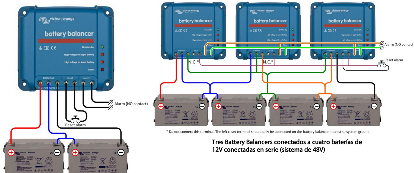
Battery Balancer conectado a dos baterías de 12V conectadas en serie (sistema de 24V)
