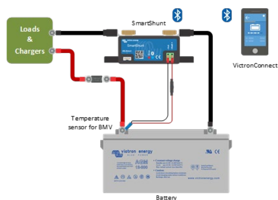
Medición de la temperatura de la batería
