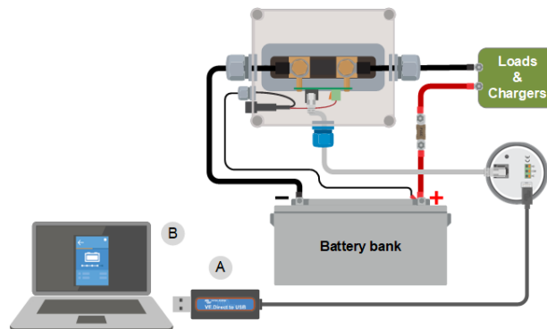
Ejemplo de conexión de una interfaz VE.Direct a USB entre el monitor de baterías y un ordenador.
