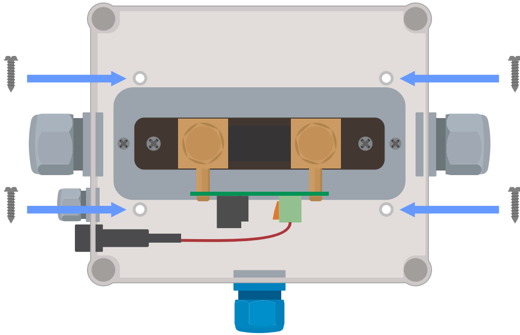
Vista superior mostrando los orificios de montaje de la carcasa del shunt.
