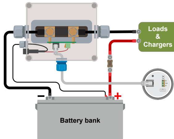
Instalación básica del monitor de baterías
