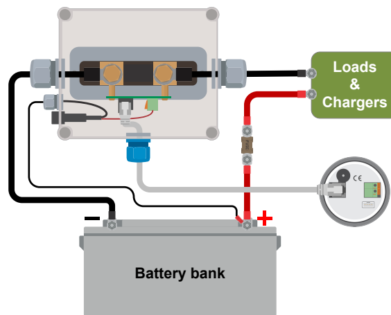
Instalación básica del monitor de baterías
