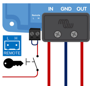
Diagrama de conexión de la anulación de la detección del apagado del motor
