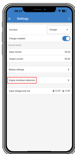
Desactivación de la detección del apagado del motor
