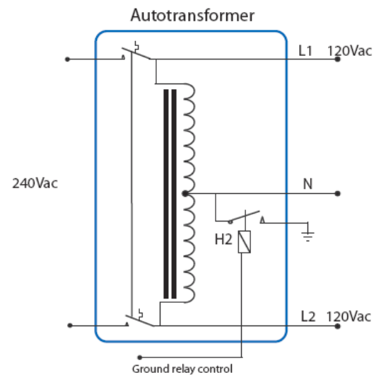
Autotransformador: diagrama esquemático
