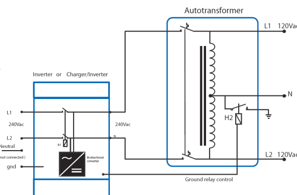
Figura 1: Alimentación de energía con fases separadas para cargas desequilibras (Debería utilizarse un transformador con relé de puesta a tierra incorporado)
