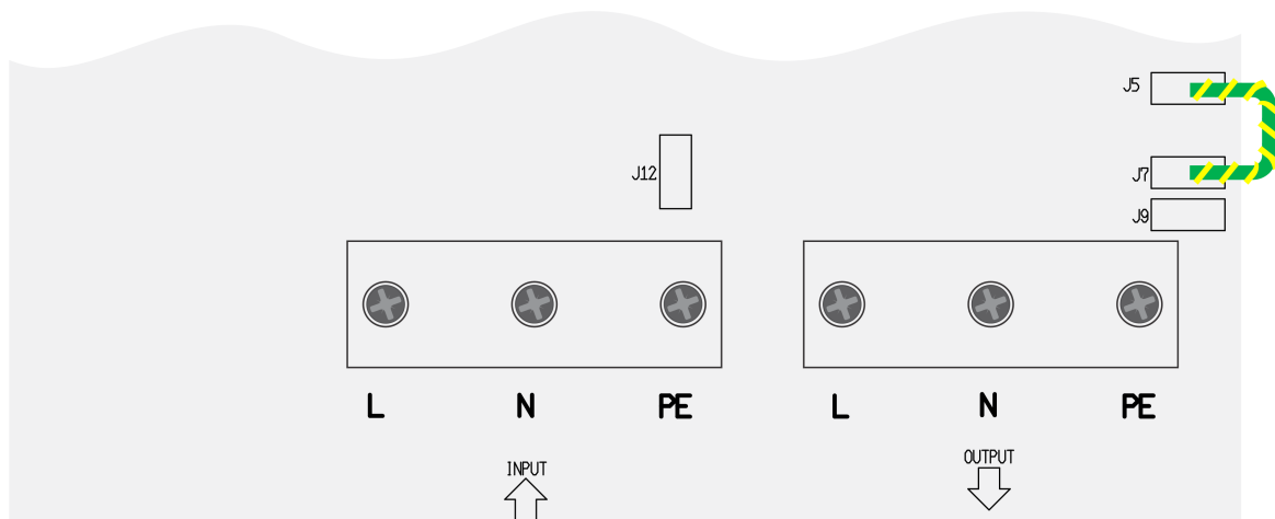
Enlace del neutro de la salida CA (N) a tierra (PE).
