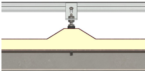
Tornillo suspensión
