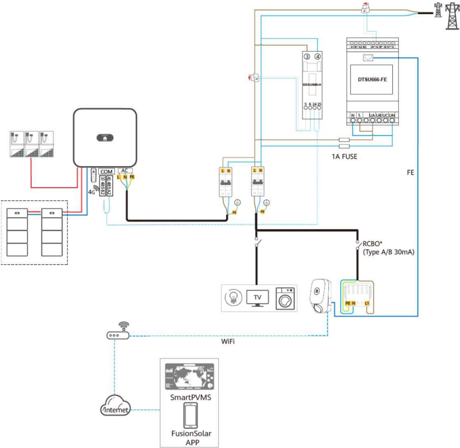
Figura 3-8 Diagrama de cableado del sistema monofásico (monofásico TN y TT)
