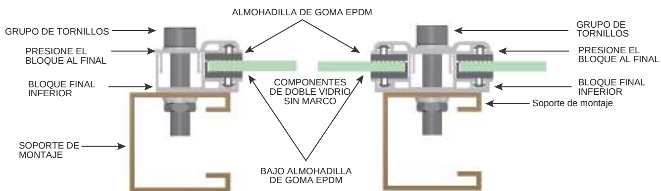
Módulo de doble vidrio de doble cara sin marco
