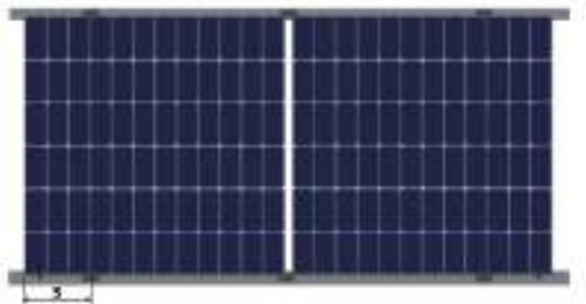
Instalación de módulo enmarcado con accesorios de fijación en lados largos. (haz paralelo a los lados largos)(longitud de la abrazadera \geq 40 mm)
