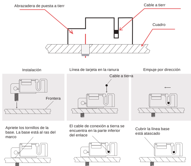
Figura 11 Método de instalación de la abrazadera de conexión a tierra Nota: La imagen de arriba usa TYCO.1954381-1 (recomendado)
