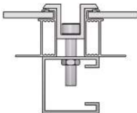
Componente de doble vidrio doble cara enmarcado
