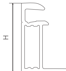
Instalación de módulo enmarcado con accesorios de fijación en lados largos. (haz perpendicular a los lados largos)(longitud de la abrazadera \geq 40 mm)
