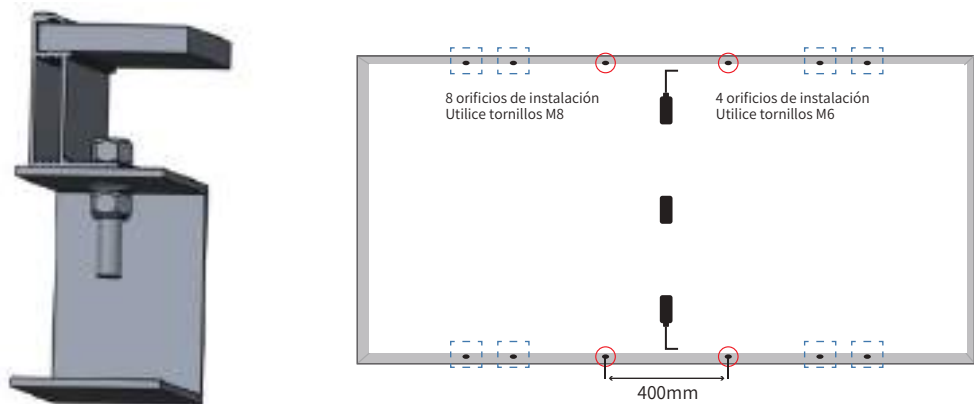
Figura 4 Diagrama de instalación del orificio de montaje del módulo de un solo lado
