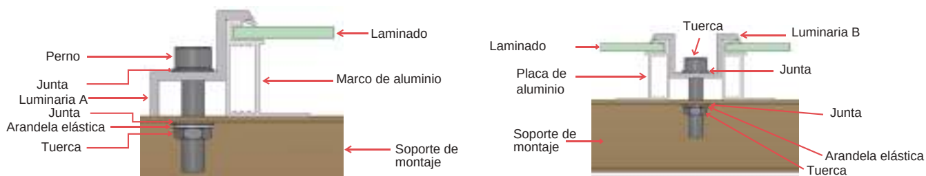
Figura 5 Diagrama de instalación del accesorio de componente de un solo lado
