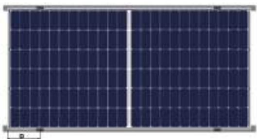
Instalación de módulo enmarcado con accesorios de fijación en lados largos. (haz paralelo a los lados largos)(longitud de la abrazadera \geq 40 mm)
