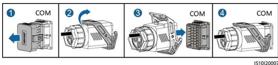
Figura 5-36 Cómo ajustar el conector del cable de señal
