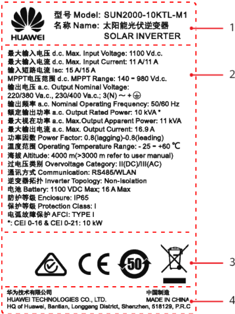
Figura 2-5 Placa de identificación (se utiliza el SUN2000-10KTL-M1 a modo de ejemplo)
