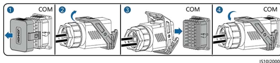
Figura 5-33 Fijación del conector del cable de señal
