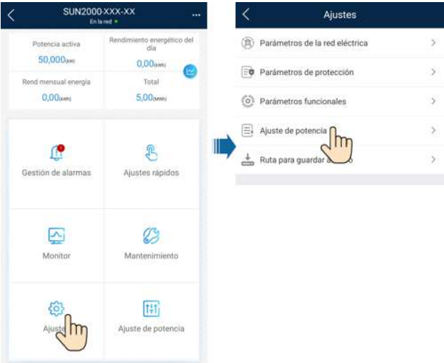
Figura 7-11 Control de potencia aparente
