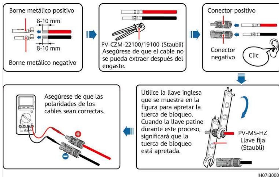
Figura 5-13 Instale los cables de entrada de CC
