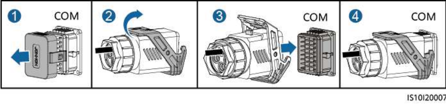
Figura 5-38 Fijación del conector del cable de señal
