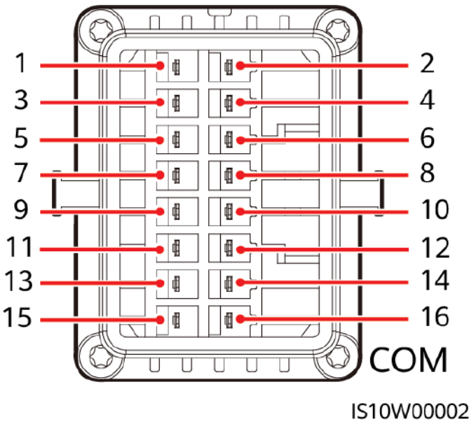
Figura 5-18 Definición de pines
