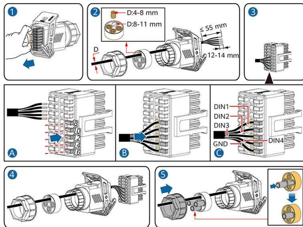
Figura 5-35 Instalación del cable
