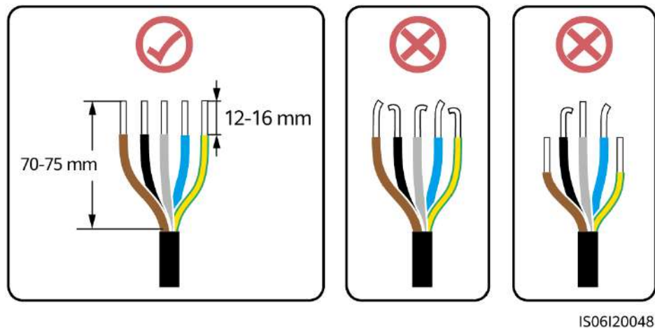
Figura 5-4 Requisitos para pelar cables
