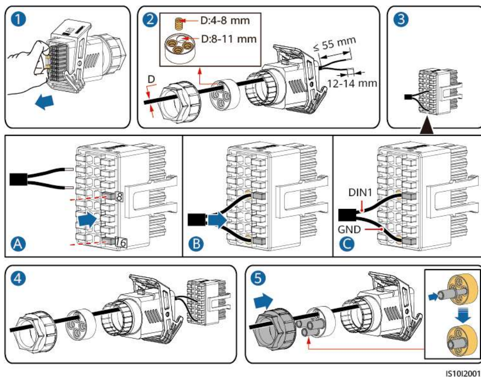
Figura 5-37 Instalación del cable
