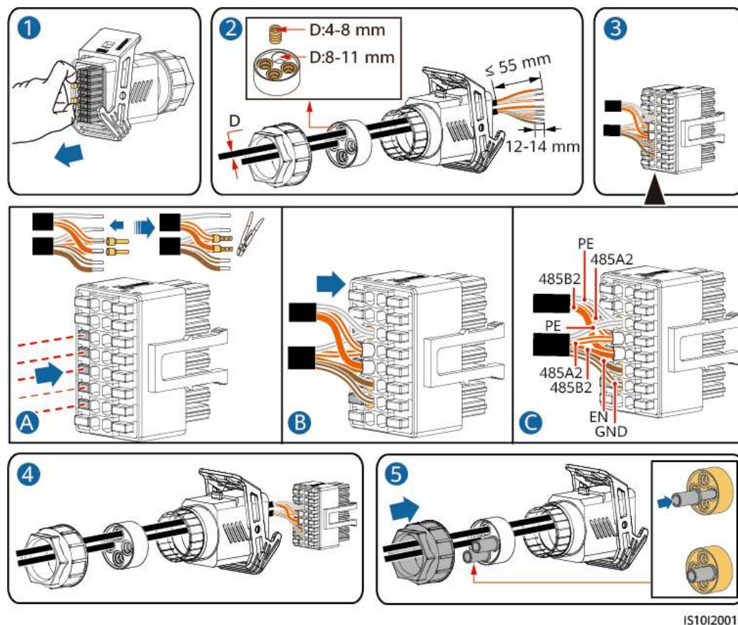
Figura 5-32 Instalación del cable
