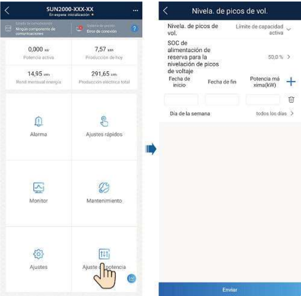
Figura 7-14 Configuración de los parámetros de control de capacidad
