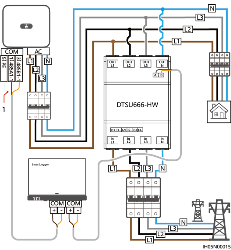
Figura 5-29 Conexión directa y trifásica de cuatro hilos (conexión en red del SmartLogger)
