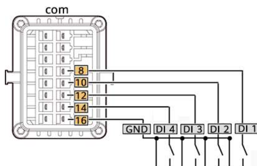
Figura 5-34 Conexión de cables
