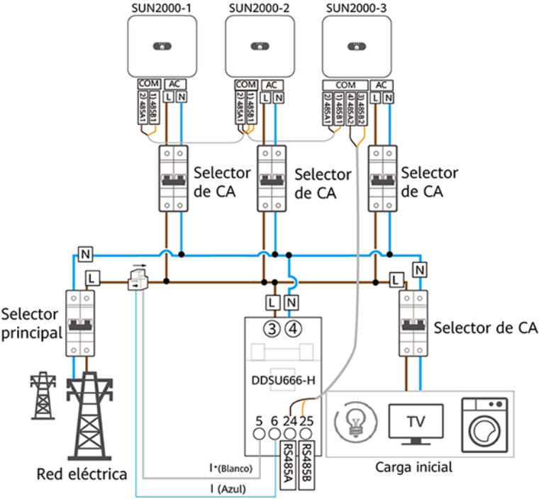
Figura 5-22 Conexión de los cables al medidor de potencia (conexión a red eléctrica en fase)
