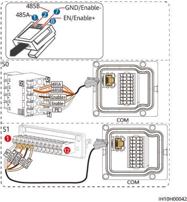
Figura 5-39 Conexión de los cables
