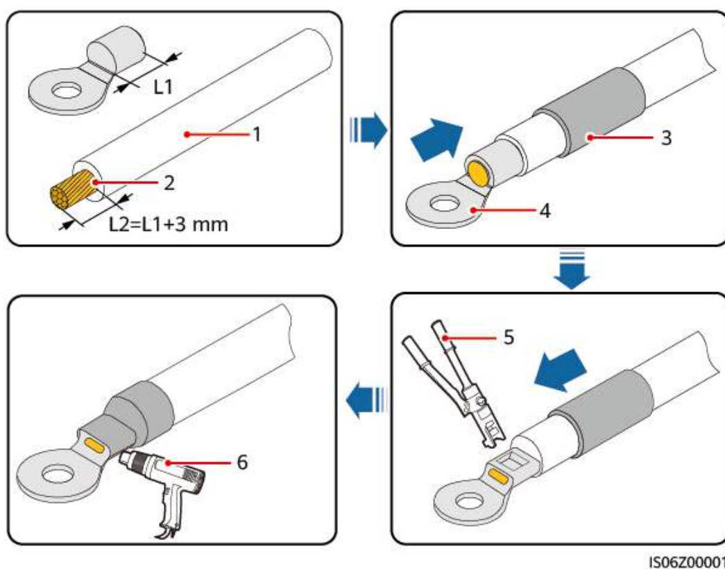
Figura 5-2 Engaste de un borne OT
