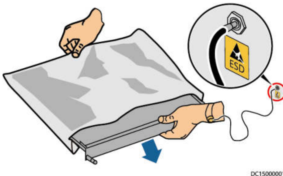
Figura 1-2 Uso de una pulsera antiestática
