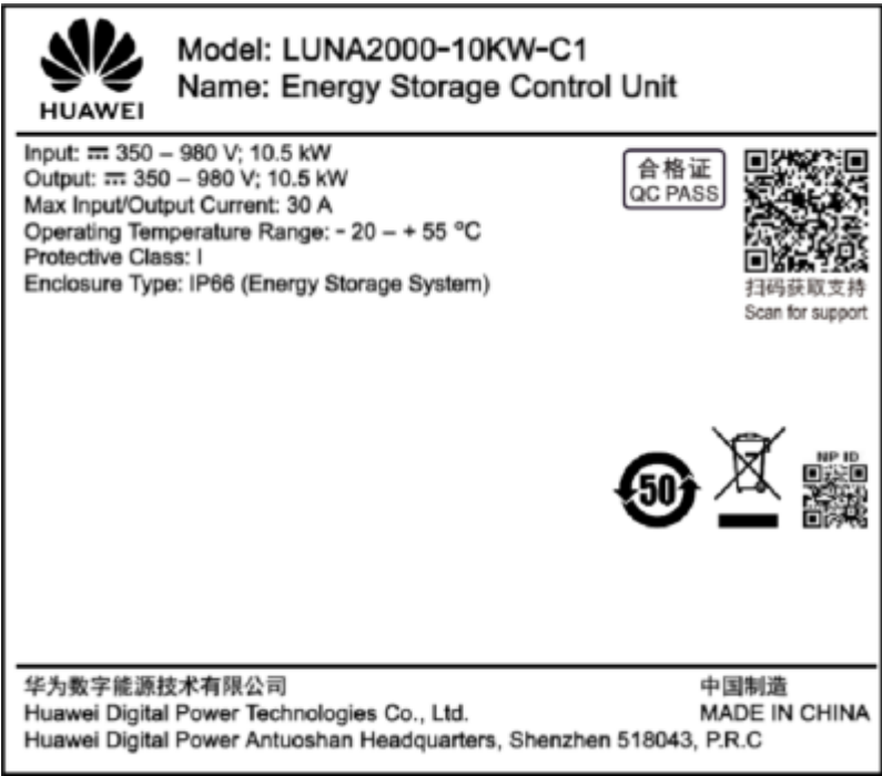
Figura 2-11 Placa de identificación de la unidad de control de almacenamiento de energía
