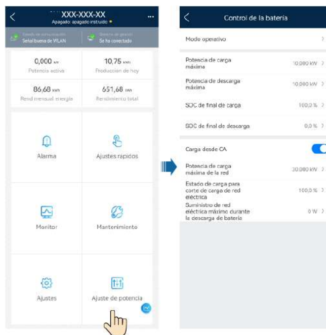
Figura 6-11 Configuración de los parámetros de control de la batería
