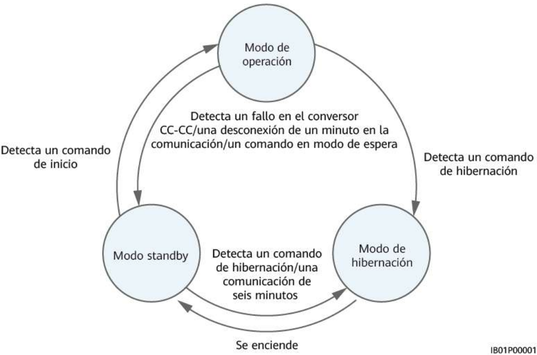
Figura 2-11 Alternancia entre modos operativos
