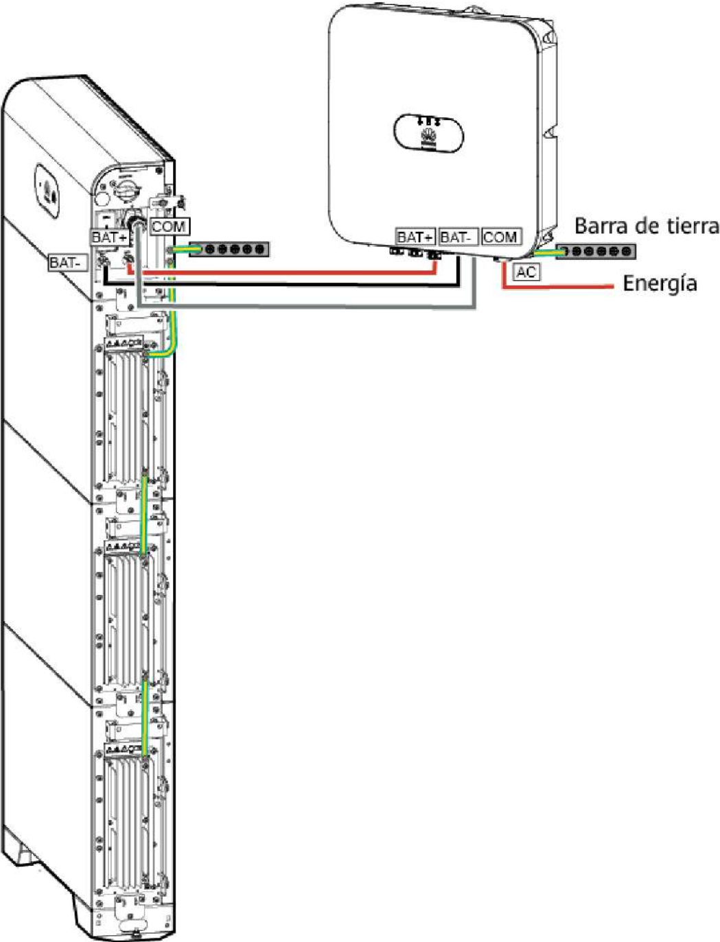
Figura 7-3 Diagrama de conexión de cables
