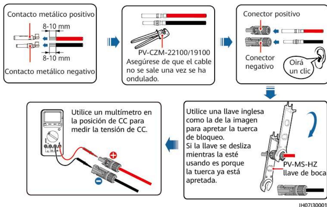
Figura 5-11 Montaje de los conectores de CC
