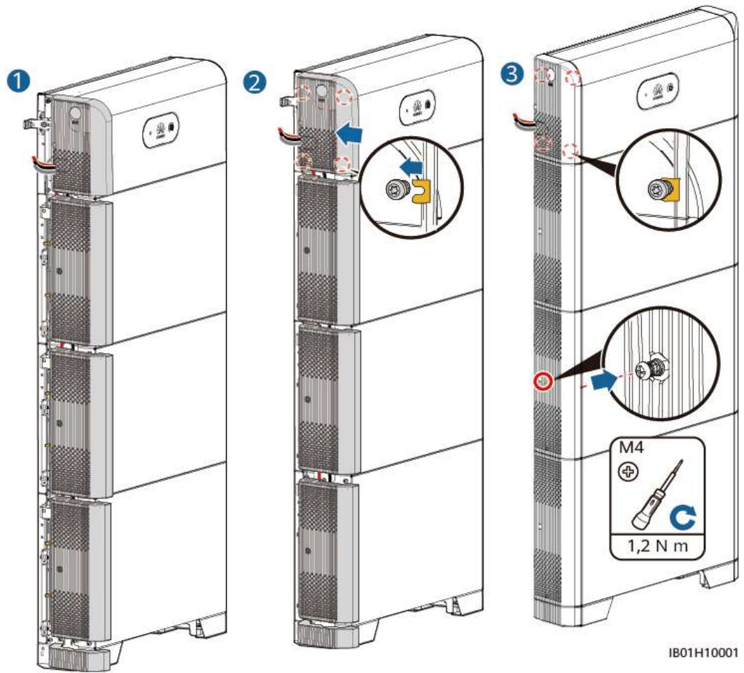
Figura 5-19 Instalación de la cubierta
