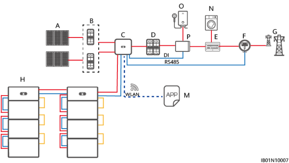
Figura 5-1 Conexión del cable de la batería
