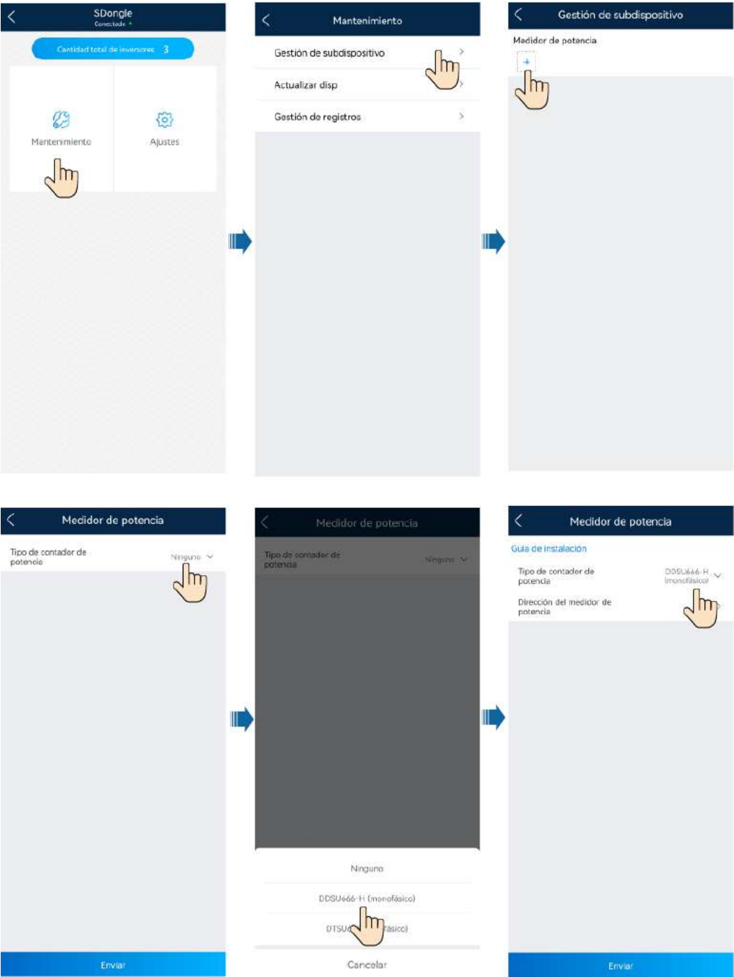
Figura 6-7 Añadidura de un contador de potencia a través del Smart Dongle
