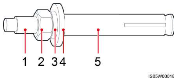
Figura 4-3 Diagrama de estructura del perno de expansión M6
