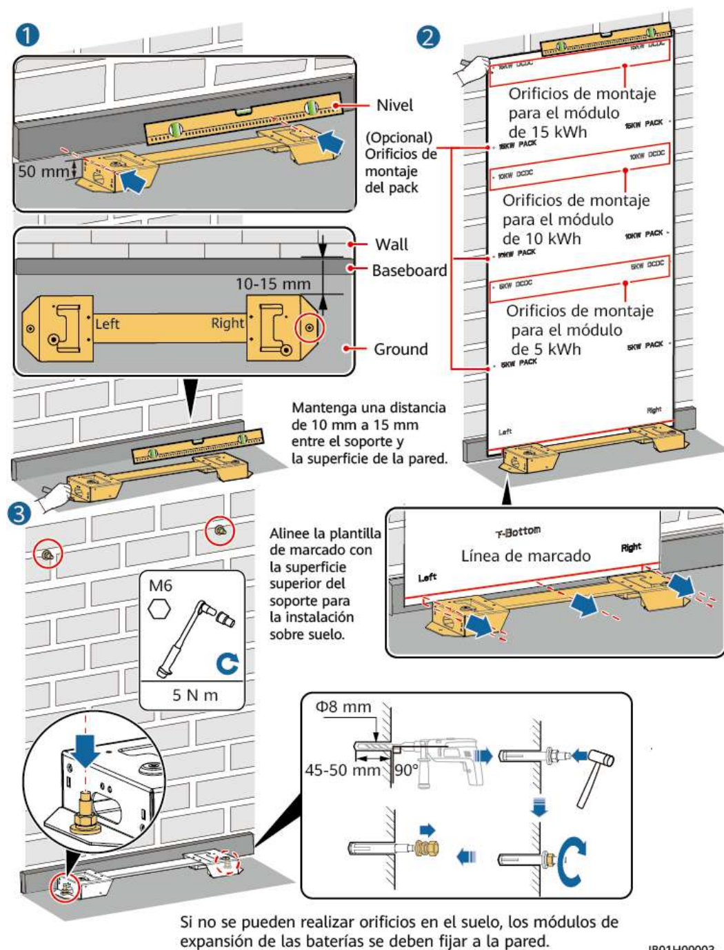
Figura 4-4 Instalación de los pernos de expansión
