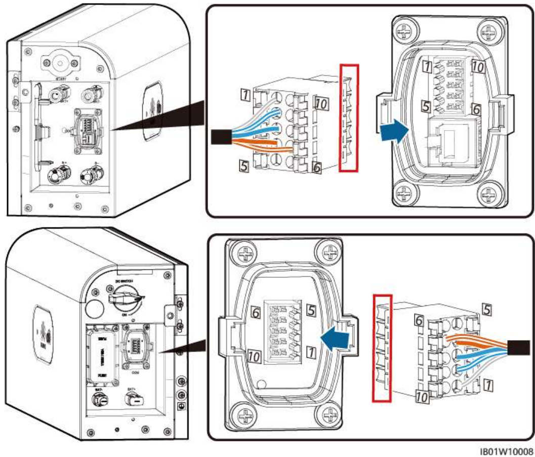
Figura 5-14 Cómo insertar el borne
