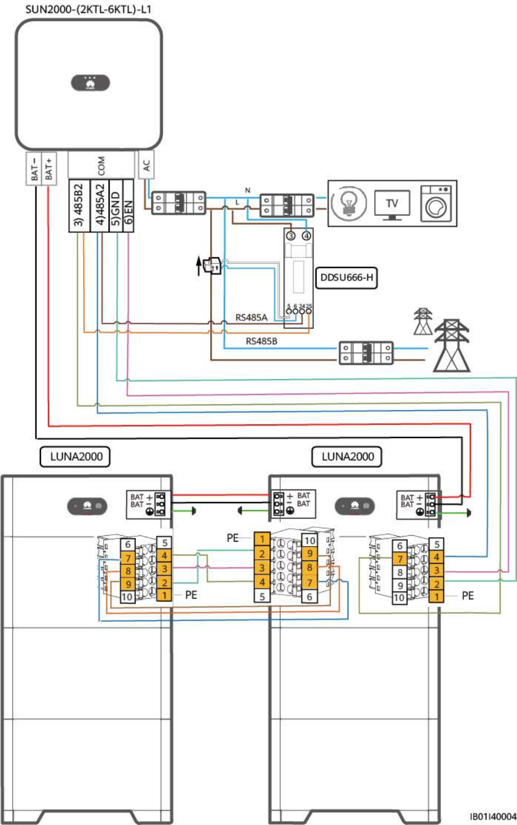
Figura 5-6 SUN2000-(2KTL-6KTL)-L1
