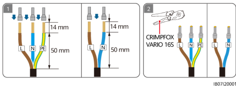
Figura 5-21 Engaste de los bornes de extremo de conductores de CA (conexión de un solo cable de fase L/N)
