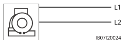
Figura 5-8 Conexión dos cables de fase L1/L2 del generador
