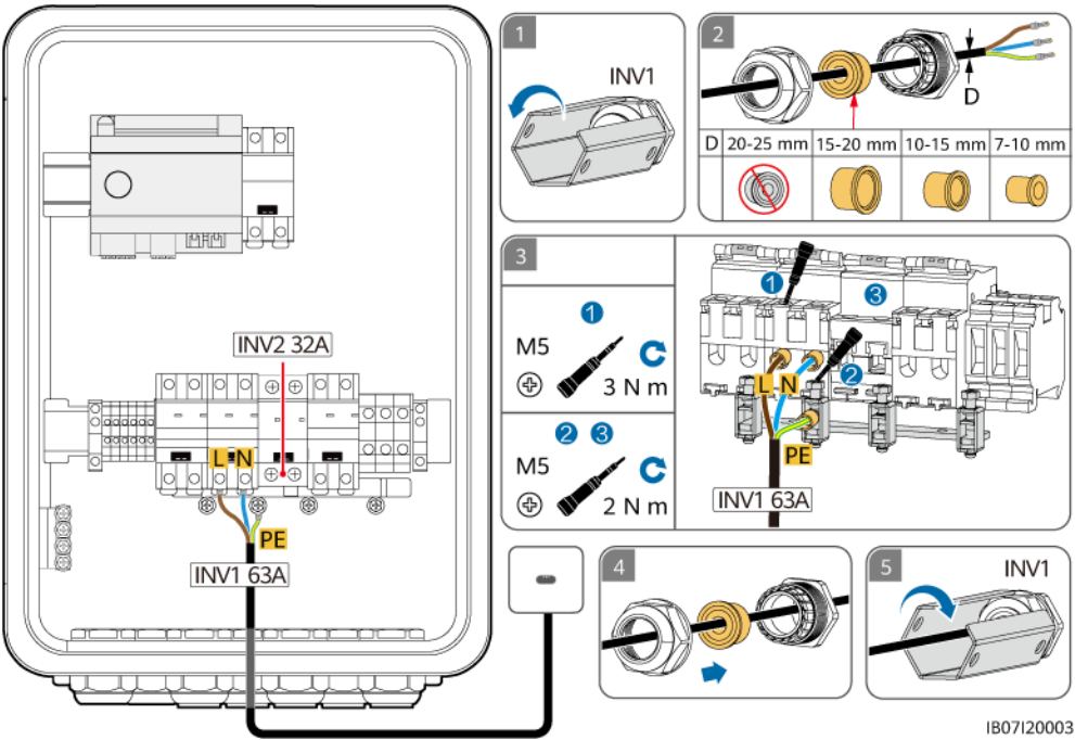
Figura 5-15 Conexión del cable de entrada de CA del inversor (conexión de un solo cable de fase L/N)
