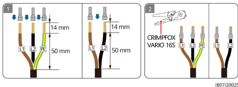
Figura 5-22 Engaste de los bornes de extremo de conductores de CA (conexión de dos cables de fase L1/L2)
