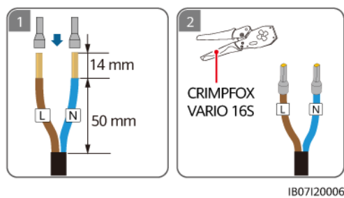
Figura 5-18 Engaste de los bornes de extremo de conductor de CA del SmartGuard-63A-AUS0
