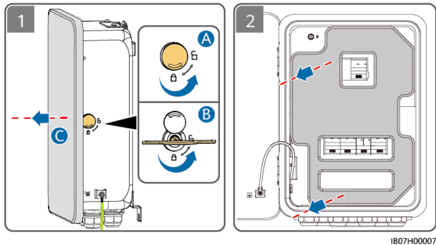
Figura 5-5 Apertura de la puerta del compartimento de mantenimiento
