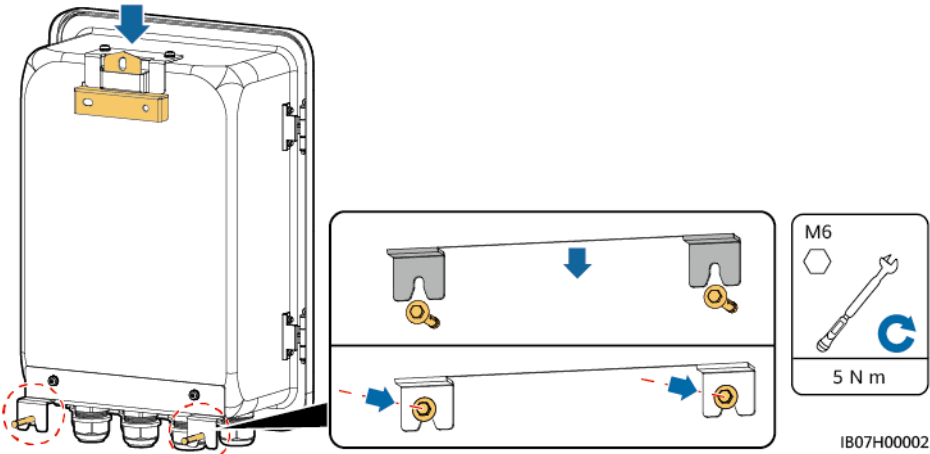
Figura 4-6 Instalación del SmartGuard
