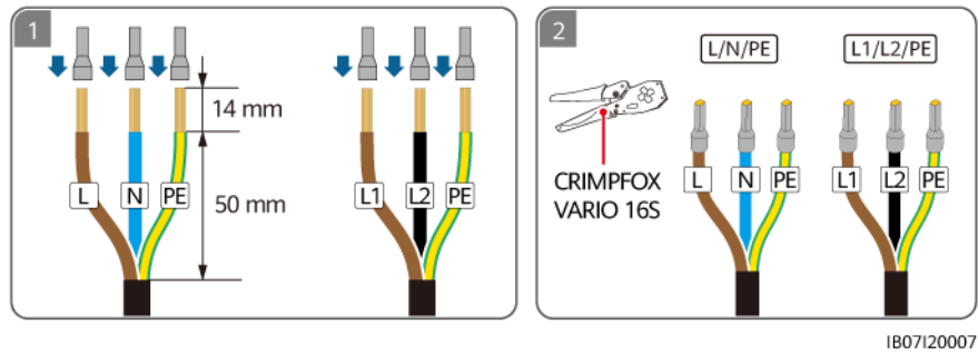
Figura 5-17 Engaste de los bornes de extremo de conductor de CA del SmartGuard-63A-S0
