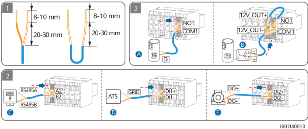
Figura 5-29 Conexión del cable de señal al borne de 14 pines
