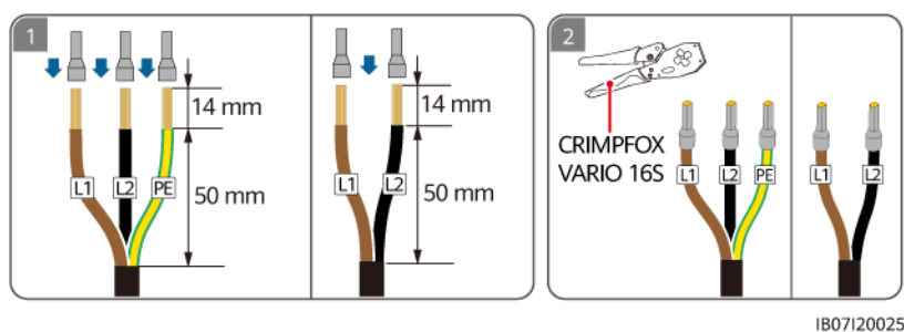
Figura 5-10 Engaste de los bornes de extremo de conductores de CA (conexión de dos cables de fase L1/L2)
