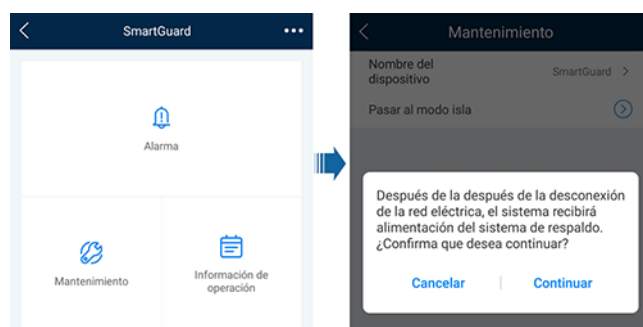
Figura 6-14 Configuración de la conmutación entre el modo con conexión a la red eléctrica y el modo isla
