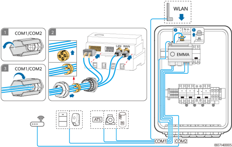
Figura 5-32 Conexión de los cables de señal del EMMA (los recuadros de rayas pequeñas indican los componentes opcionales)
