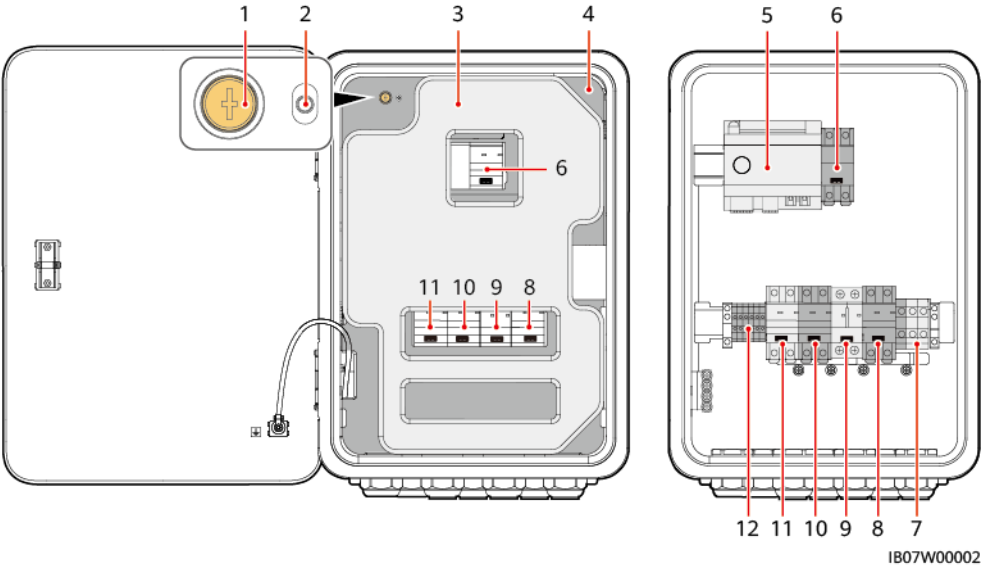
Figura 2-10 Compartimento de mantenimiento y bornes de cableado
