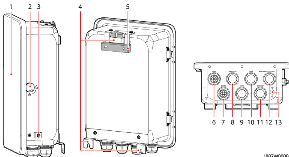
Figura 2-9 Aspecto y puertos
