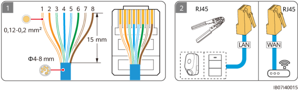
Figura 5-31 Cable de comunicaciones FE (los recuadros de rayas pequeñas indican los componentes opcionales)
