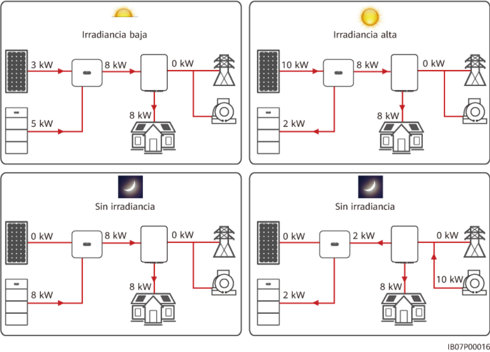
Figura 2-6 Ilustración de la potencia máxima en modo isla
