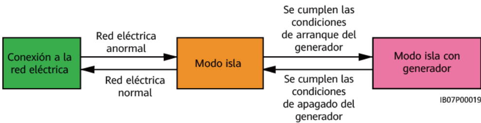
Figura 2-12 Modos de funcionamiento
