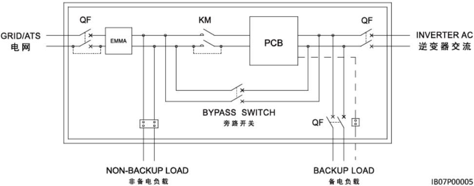
Figura 2-11 Diagrama eléctrico del SmartGuard
