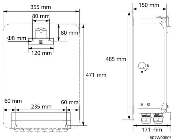
Figura 4-1 Dimensiones de la ménsula de montaje
