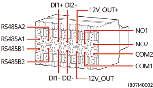
Figura 5-28 Definiciones de los pines
