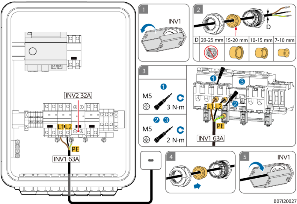
Figura 5-16 Conexión del cable de entrada de CA del inversor (conexión de dos cables de fase L1/L2)
