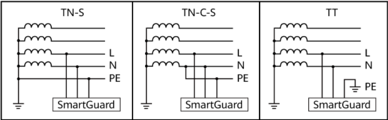
Figura 2-7 Sistema de puesta a tierra (conexión de un solo cable de fase L/N)
