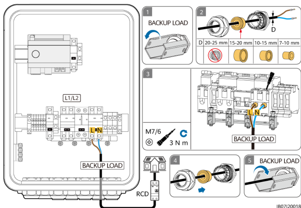
Figura 5-20 Conexión del cable de alimentación de salida de las cargas con respaldo del SmartGuard-63A-AUS0
