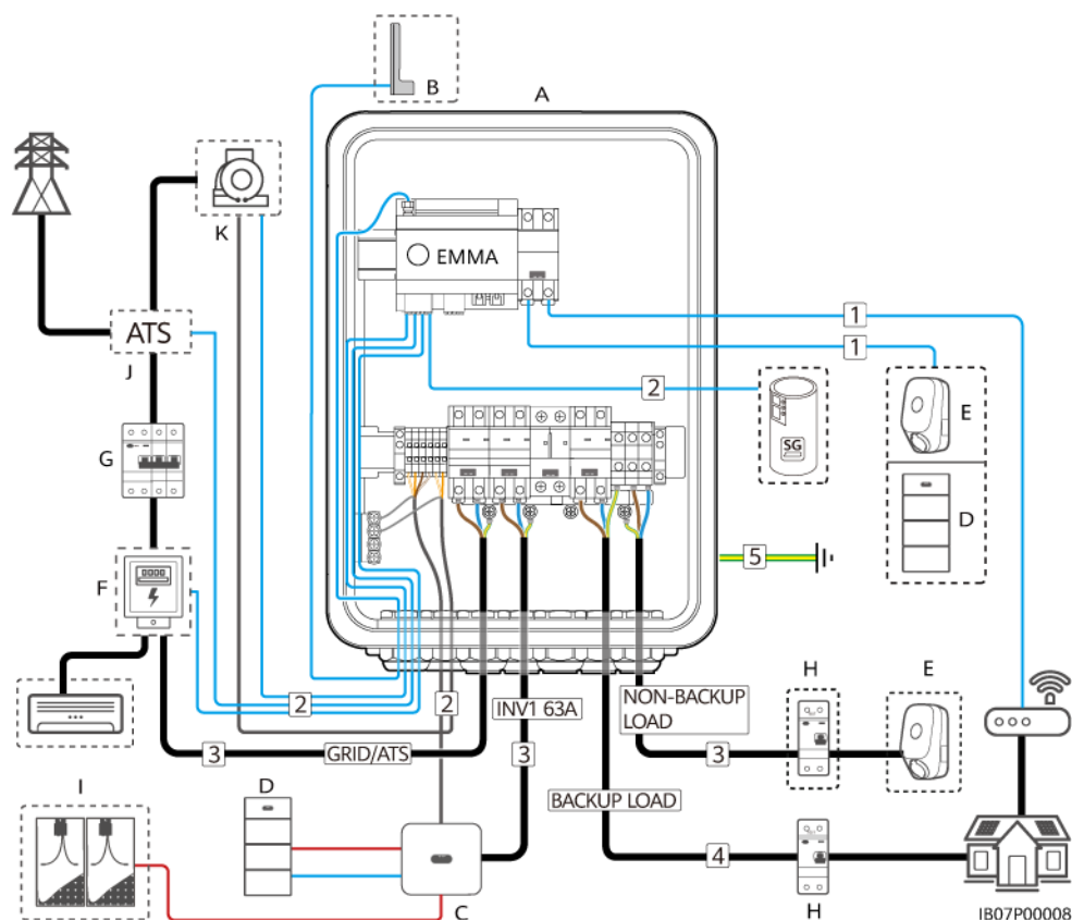
Figura 5-1 Conexiones de los cables (los cuadros de rayas pequeñas muestran la configuración opcional)
