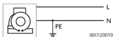
Figura 5-7 Conexión a tierra del conductor neutro del generador (conexión de un solo cable de fase L/N)
