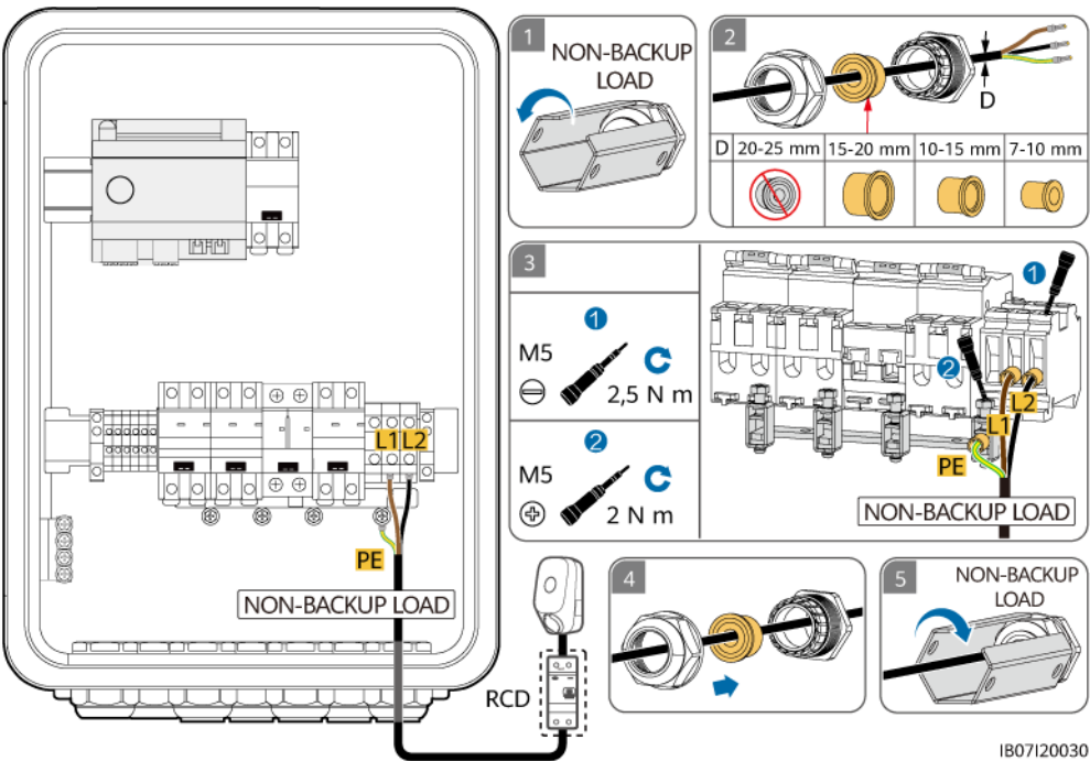
Figura 5-24 Conexión del cable de alimentación de salida de las cargas sin respaldo (conexión de dos cables de fase L1/L2)
