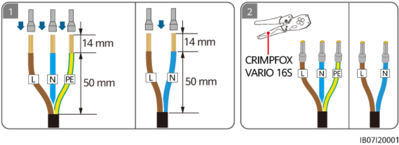
Figura 5-13 Engaste de los bornes de extremo de conductores de CA (conexión de un solo cable de fase L/N)
