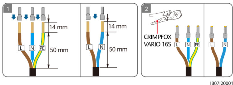
Figura 5-9 Engaste de los bornes de extremo de conductores de CA (conexión de un solo cable de fase L/N)
