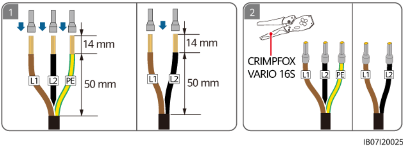
Figura 5-14 Engaste de los bornes de extremo de conductores de CA (conexión de dos cables de fase L1/L2)
