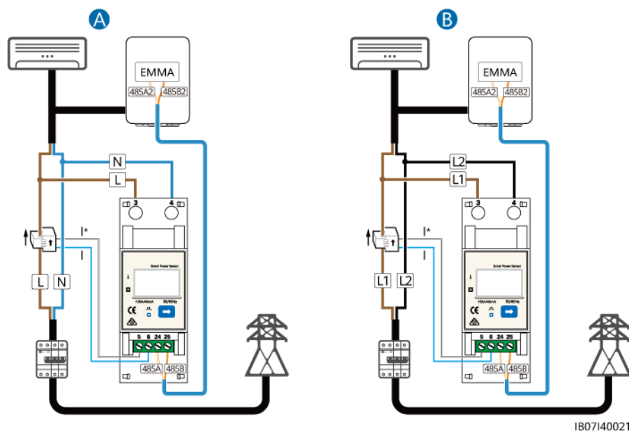
Figura 5-30 Conexión del cable de comunicaciones del medidor de potencia
