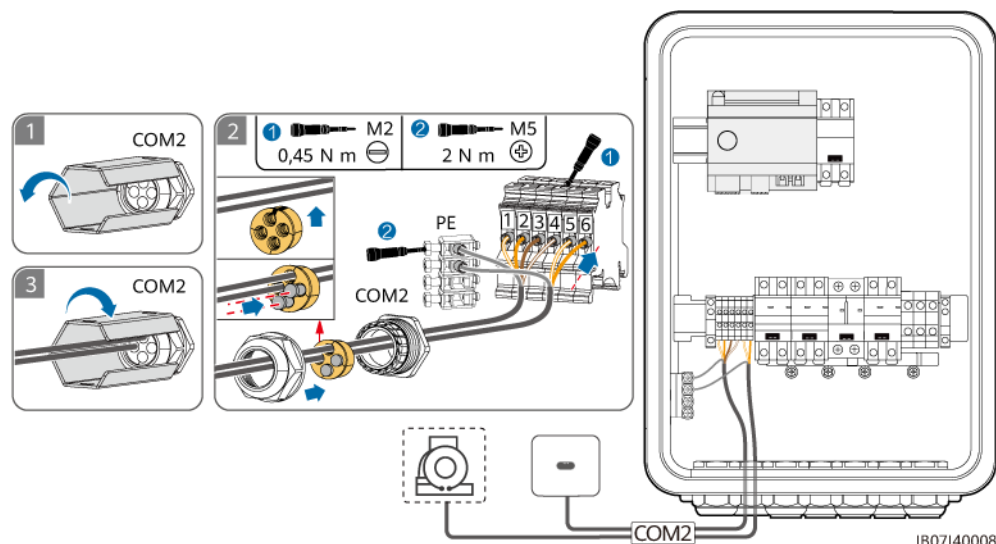
Figura 5-26 Conexión del cable de señal del SmartGuard (el recuadro de rayas pequeñas indica un componente opcional)
