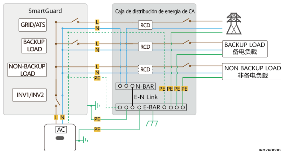
Figura 2-3 Diagrama de cableado residencial del SmartGuard-63A-AUS0 (las líneas de rayas pequeñas muestran las conexiones de cable opcionales)
