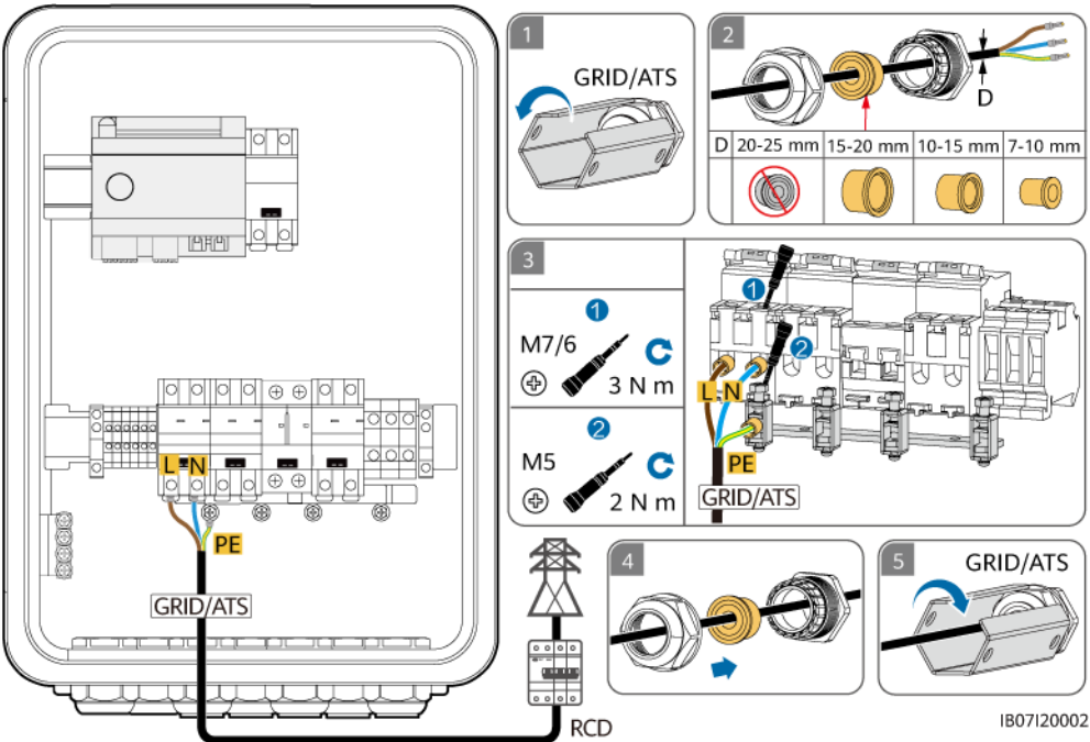
Figura 5-11 Conexión del cable de salida de CA de la red eléctrica (conexión de un solo cable de fase L/N)
