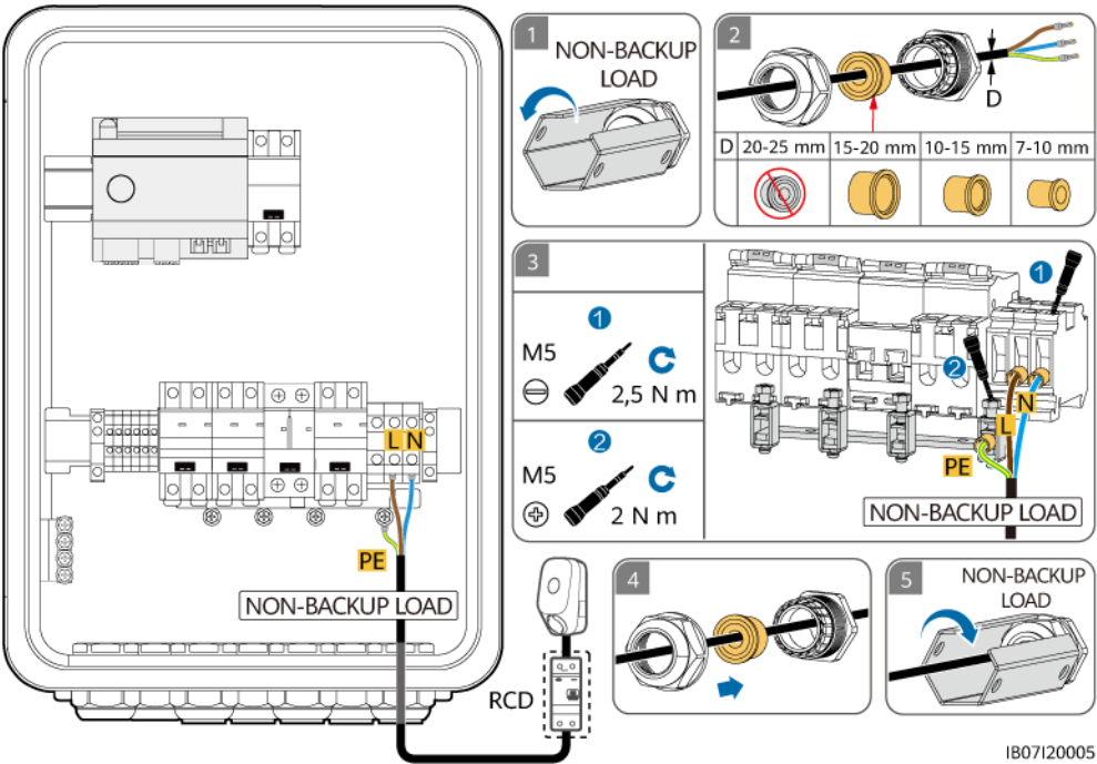
Figura 5-23 Conexión del cable de alimentación de salida de las cargas sin respaldo (conexión de un solo cable de fase L/N)
