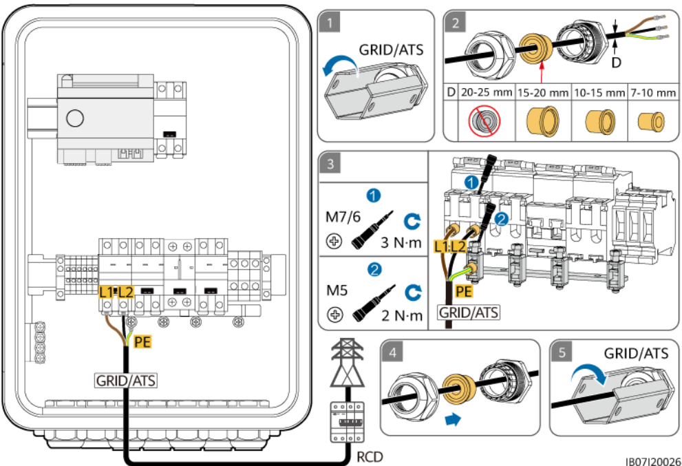
Figura 5-12 Conexión del cable de salida de CA de la red eléctrica (conexión de dos cables de fase L1/L2)
