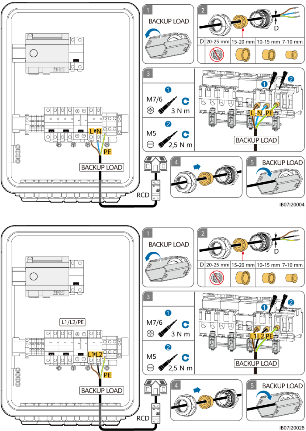
Figura 5-19 Conexión del cable de alimentación de salida de las cargas con respaldo del SmartGuard-63A-S0
