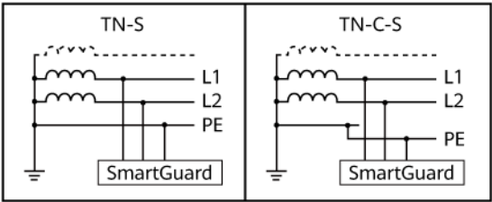
Figura 2-8 Sistema de puesta a tierra (conexión dos cables de fase L1/L2)
