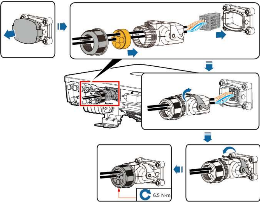
Figura 5-31 Fijación del conector del cable de señal
