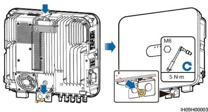
Figura 4-10 Ajuste de las tuercas
