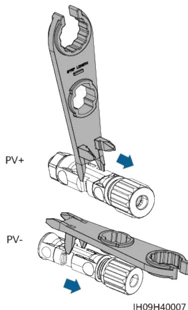
Figura 5-11 Extracción de un conector de CC
