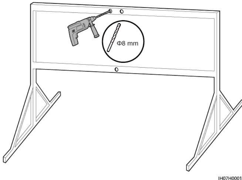
Figura 4-13 Perforación de orificios
