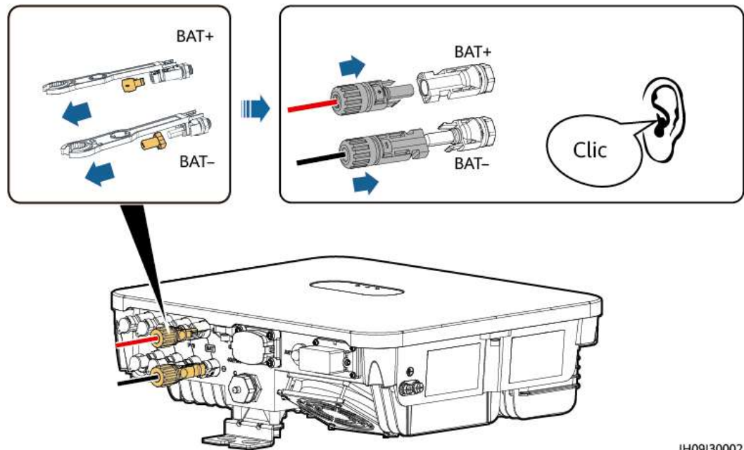
Figura 5-12 Conexión de los cables de las baterías
