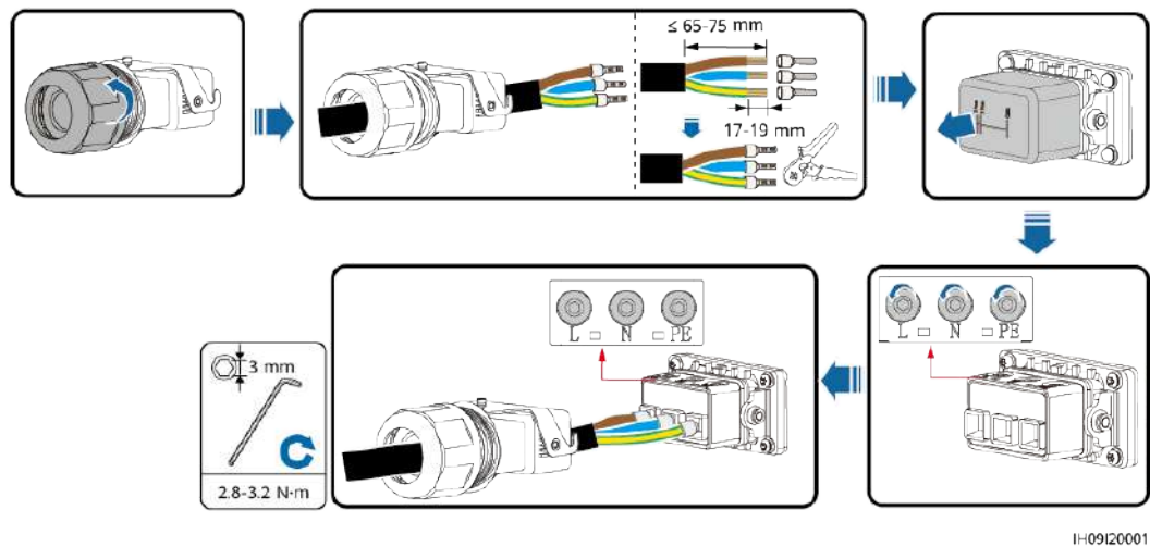
Figura 5-4 Instalación del cable de alimentación de CA
